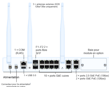
Vue arrière
